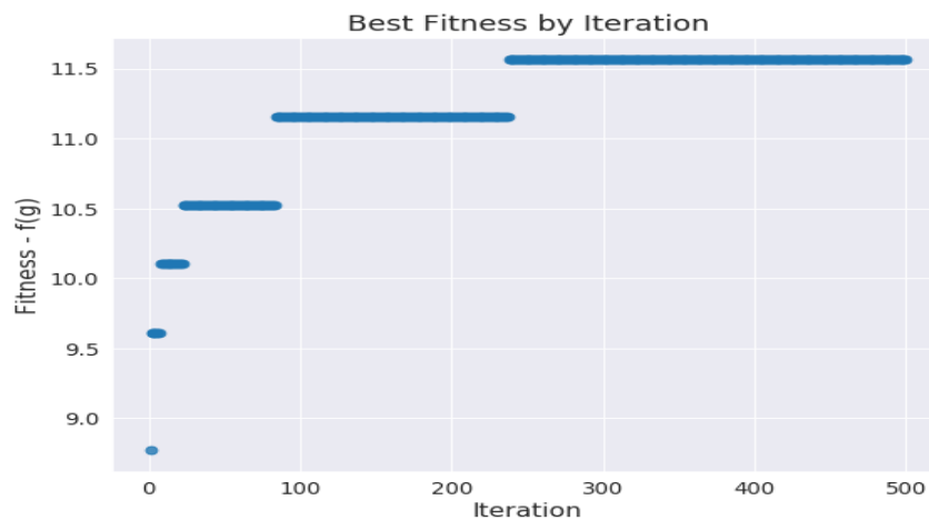
Figure.11. Best Fit Iteration
